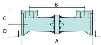
寸法図
