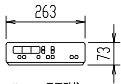
リモコン正面形状
