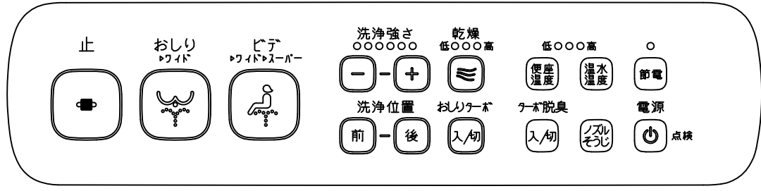
操作部拡大図
