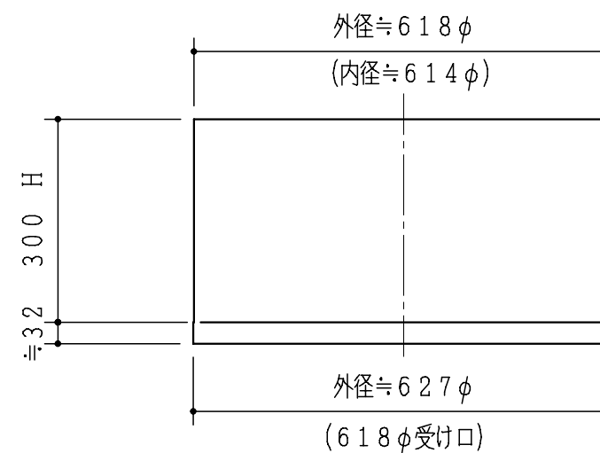
600φ×300H (FRP製)
